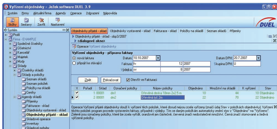
Ukázka operace vyřízení přijaté objednávky s automatickou tvorbou faktury a výdejky.
